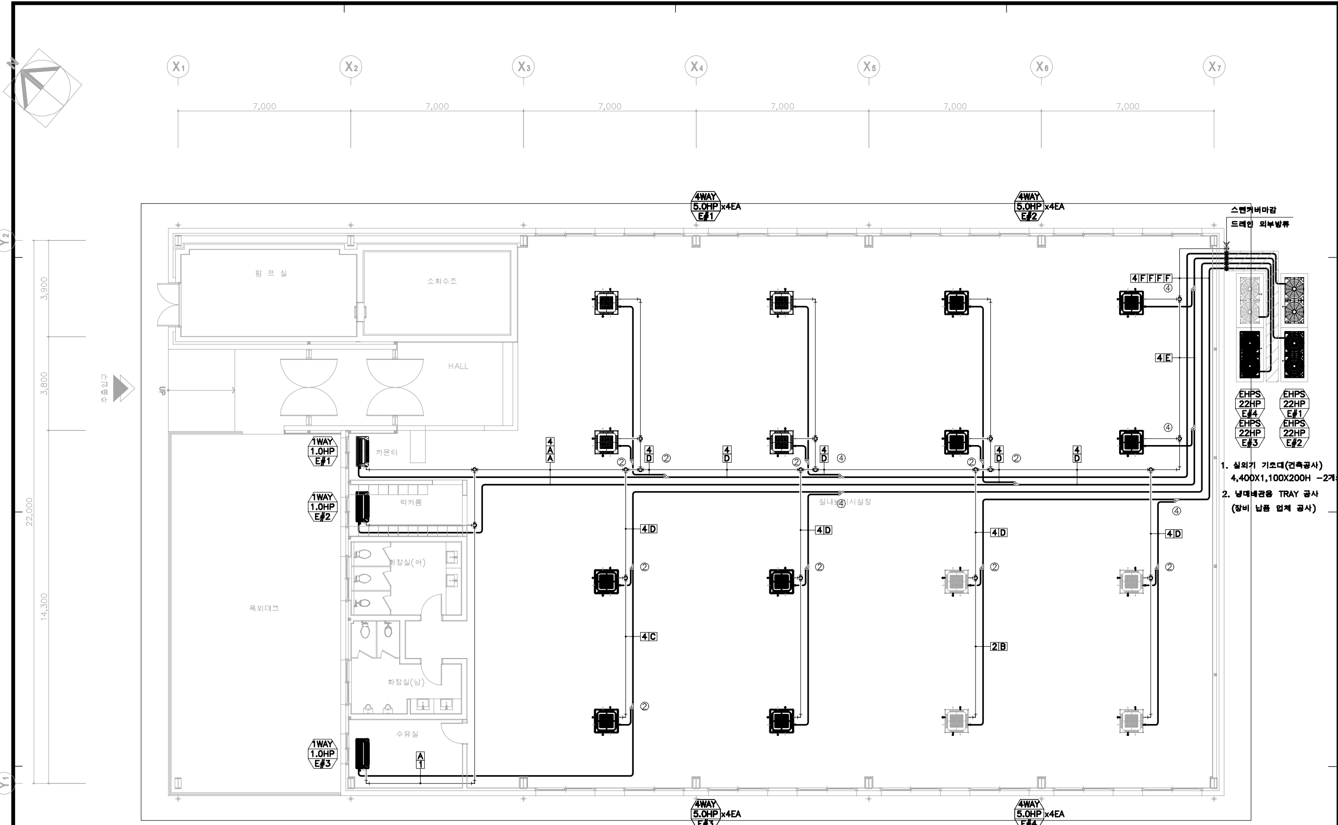
1층 냉난방 배관 평면도 SCALE A1:1/75 A3:1/150
