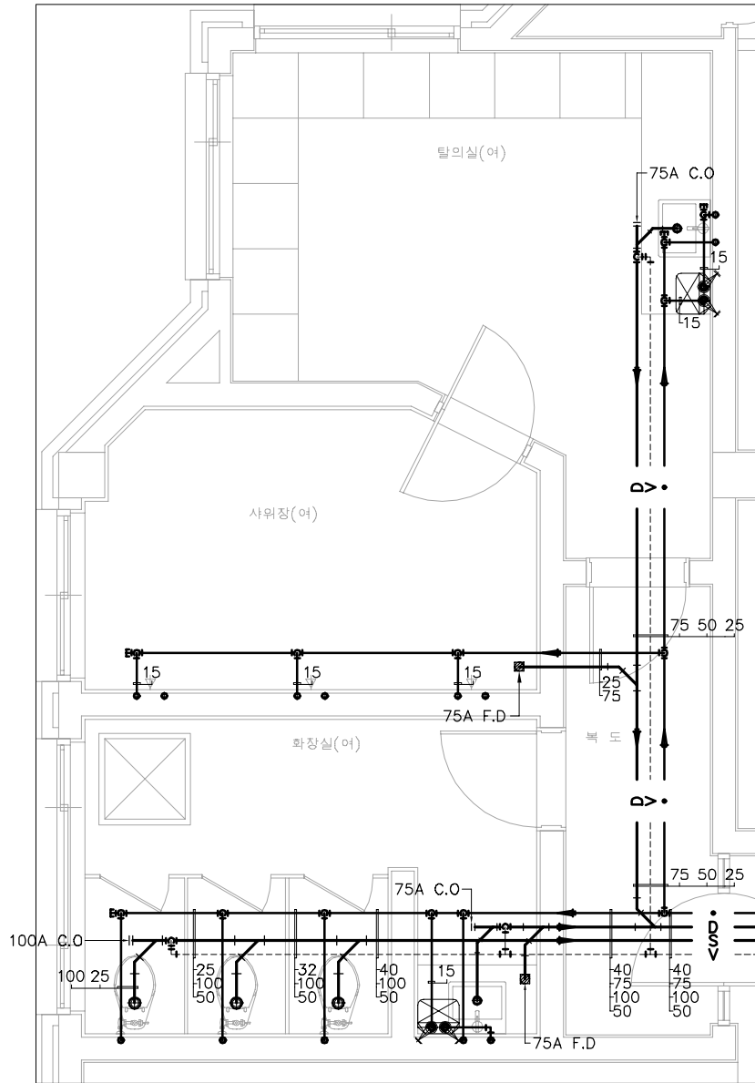
1층 위생 배관 평면도
