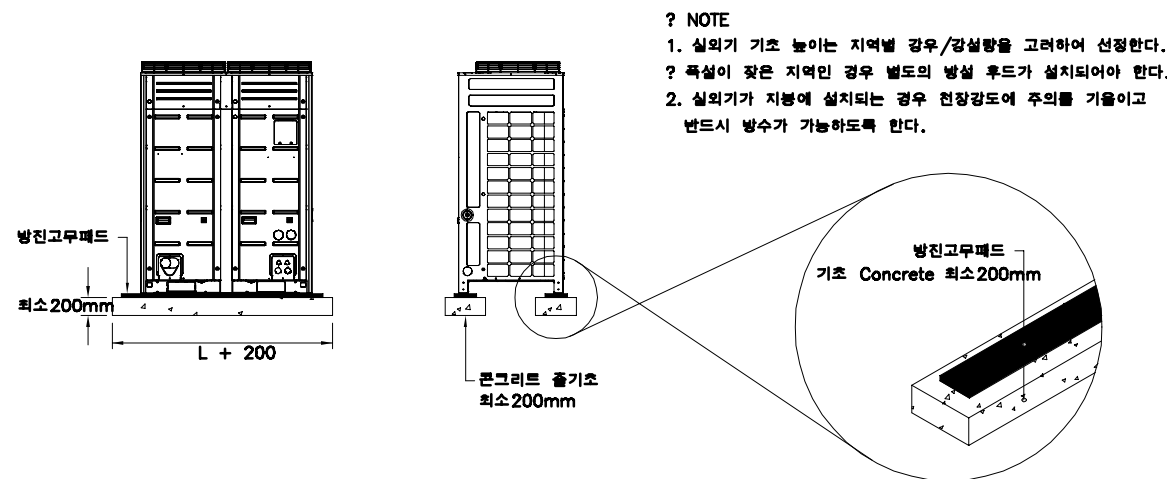
실외기 콘크리트 줄기초 상세도
