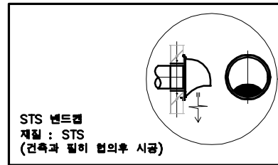
STS 밴드캡 설치 상세도
