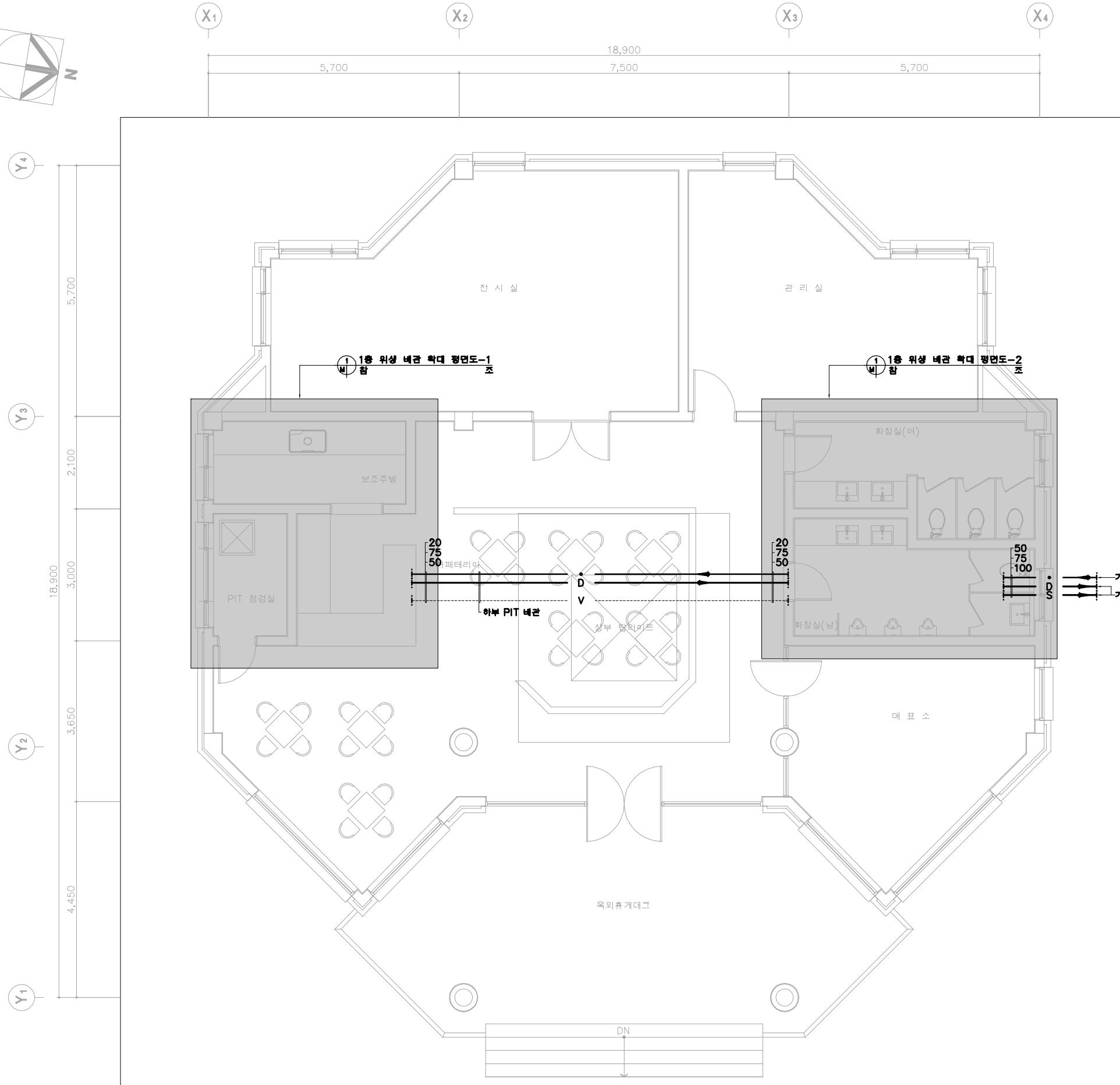
1 1층 위생 배관 평면도 SCALE A1: 1/50 A3: 1/100
