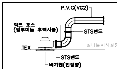
천장형 배기팬 설치 상세도
