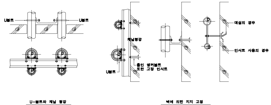
U-볼트와 채널 형강
