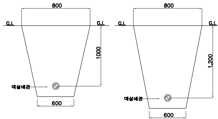
일반 관 매설 배관 상세도
