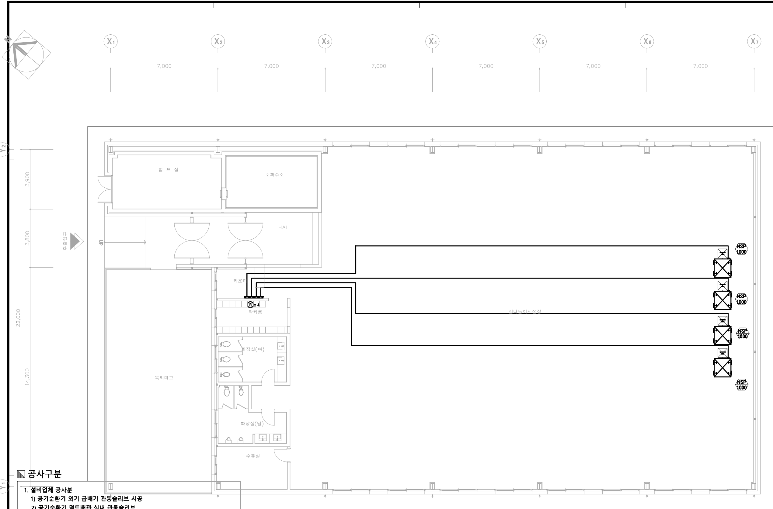
1 1층 전열교환기 제어 평면도 SCALE A1:1/75 A3:1/150
