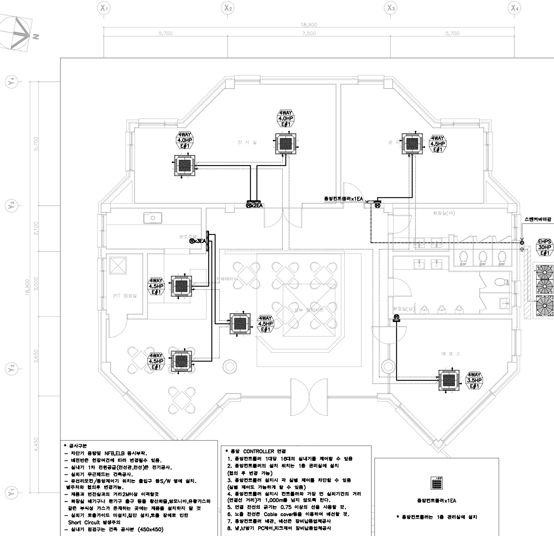
1층 냉난방 제어 평면도 SCALE A1: 1/50 A3: 1/100
