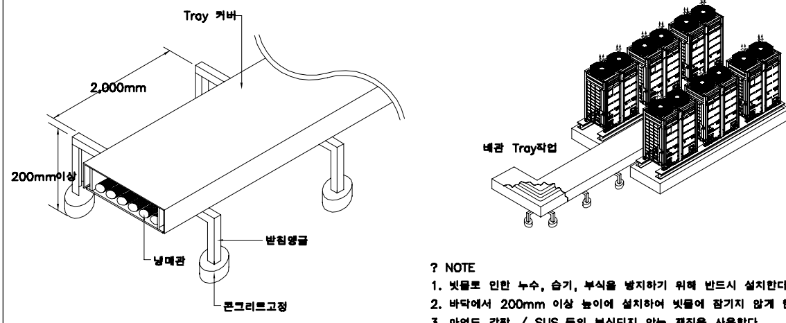
냉매배관용 TRAY 설치도
