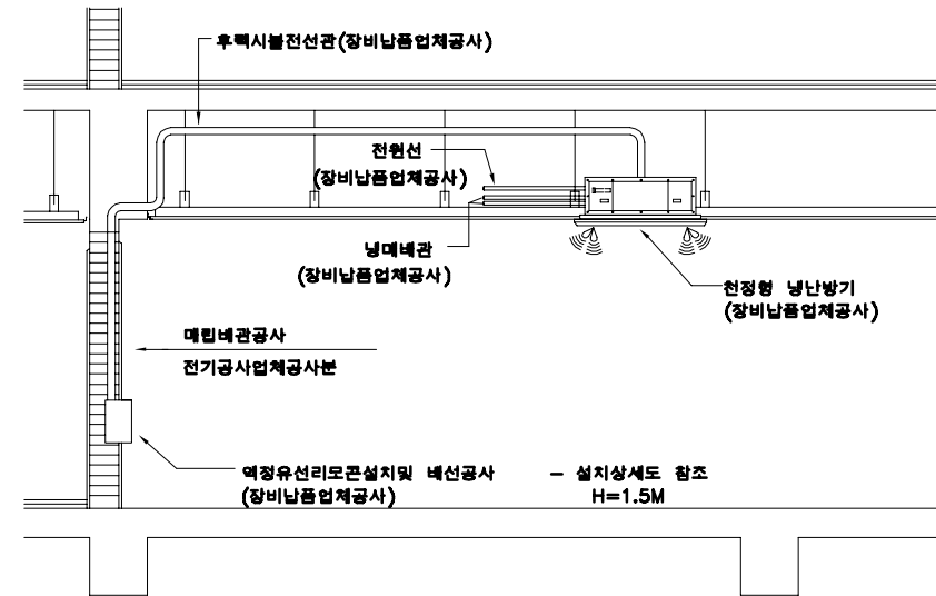
천정카세트형 냉.난방기 배관/배선 설치상세도
