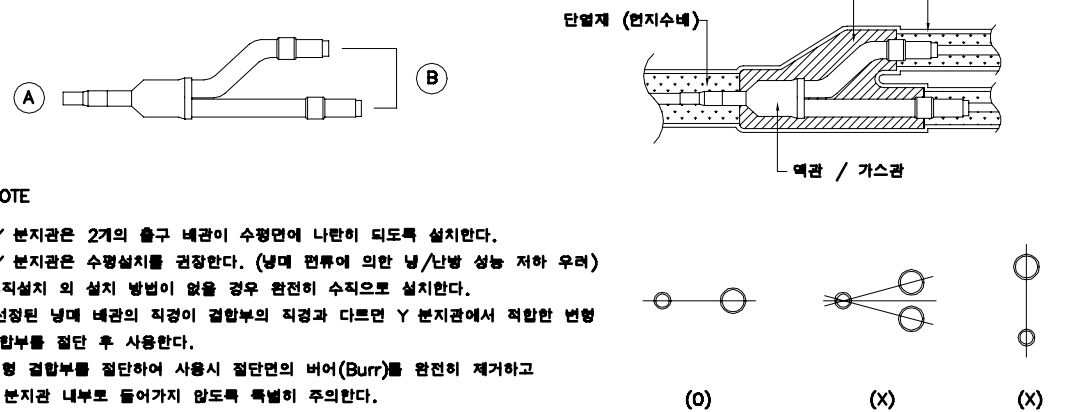
Y 분기관 상세도
